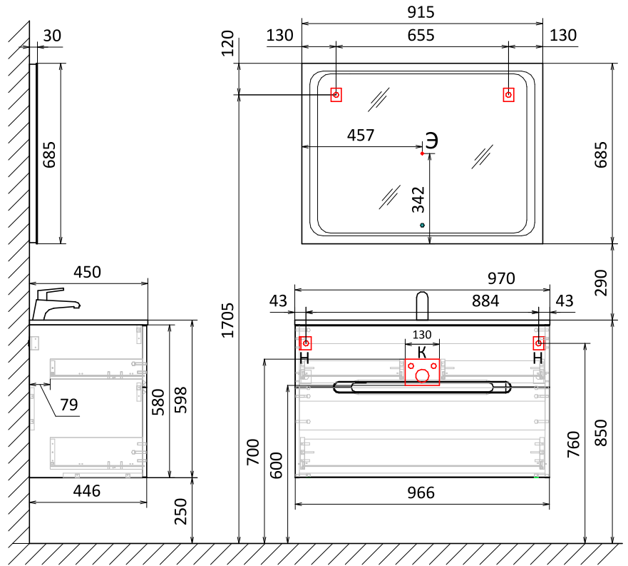
Тумба подвесная Modul 100
